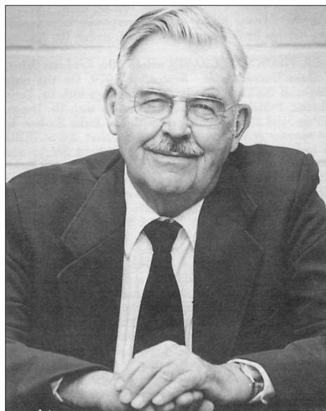
Prof. C. G. Bookhout, 1907—2003
